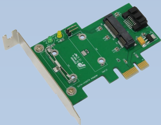
MP3S (PCIe スロット用 SATA-mSATA アダプタ) X1
