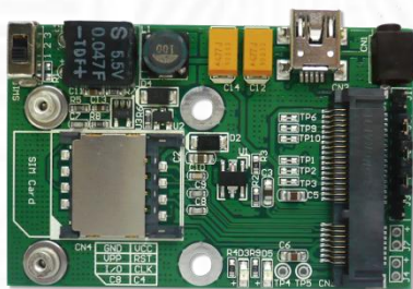
USBMI モジュール (無線通信 Mini Card 用 USB アダプタ ver1.1b) x1 * モジュールのみ。筐体はなし。
