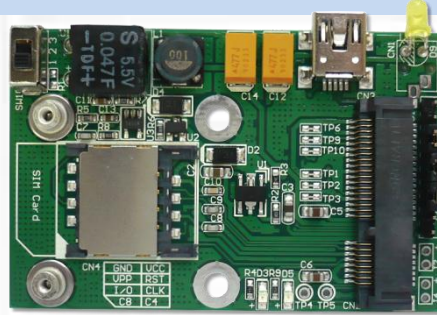
USBMIモジュール (筐体なし)
