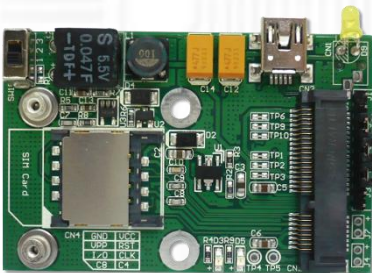
USBMI モジュール (無線通信 Mini Card 用 USB アダプタ ver1.1b) x1 * モジュールのみ。筐体はなし。
